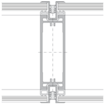
Glaselement Achsrasterfuge
