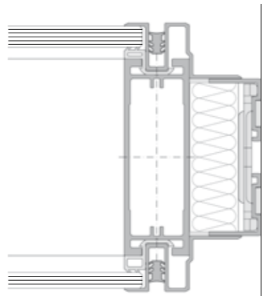
Glaselement Wandanschluss
