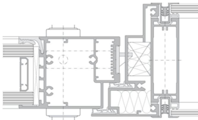
Alurahmentür Schlossseite
