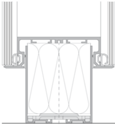
Glaselement Bodenanschluss
