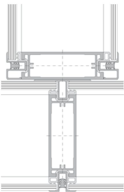
Glaselement T-Anschluss
