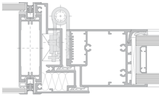
Alurahmentür Bandseite
