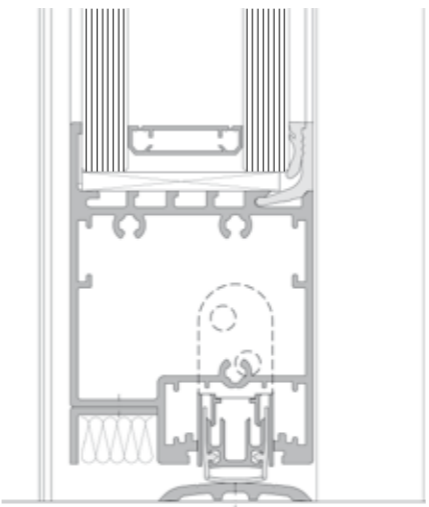
Alurahmentür Bodenanschluss
