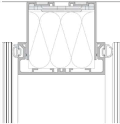
Glaselement Deckenanschluss
