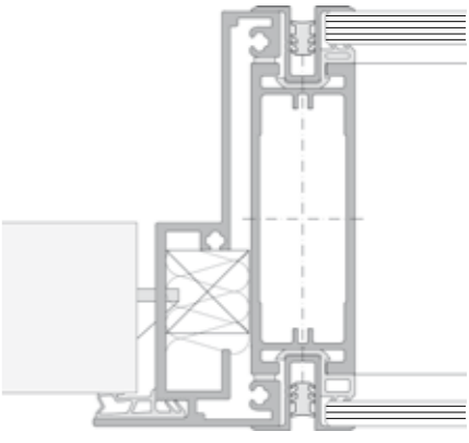
Volltürblatt Schlossseite
