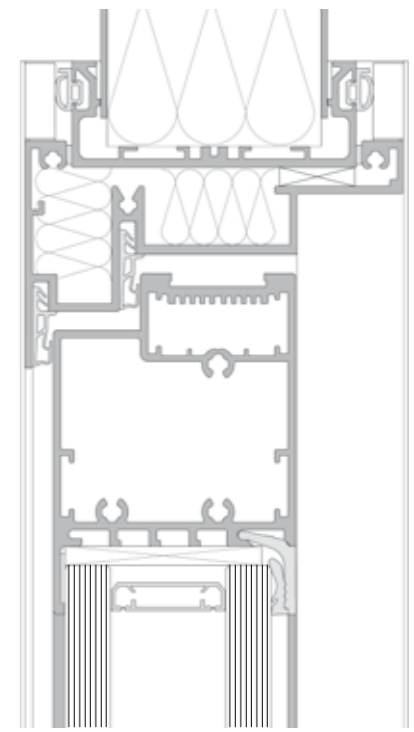
Alurahmentür Deckenanschluss
