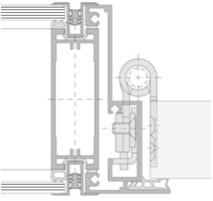
Volltürblatt Bandseite
