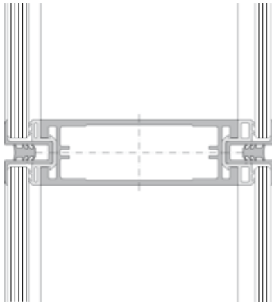
Glaselement Querfuge
